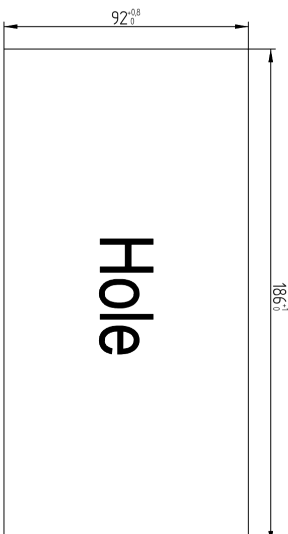
패널컷트도
